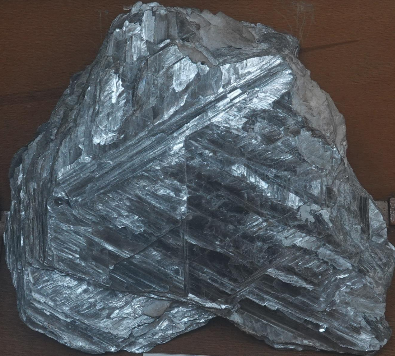
M6416 МУСКОВИ, МИКРОКЛИН, ГРАНАТ ГР. MUSCOVITE, MICROCLINE, GARNET, GR. Вищерица, Зап.Родопи, проф.В.Вергилов 1958 г.
